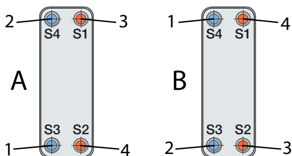
Figura 5. Circuito simple: A evaporador; B condensador.
